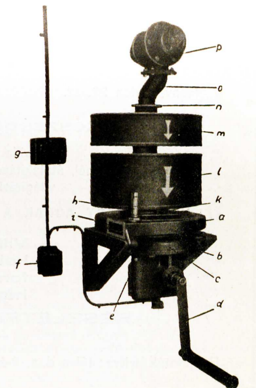
p = szívóvezeték elzáró szelepe, o = rugalmas összekötő fémcső, n = csatlakozóanya, m = füstszűrő, l = gápszűrő, k = szűrőcsatlakozó rész, a = ventilátor, b = faligám, c = hajtómű, d = kéziforgattyú, e = elektromotor, f = elektromos kapcsoló, g = biztosító, h = levegőmennyiségmérő, i = fojtószelep.
