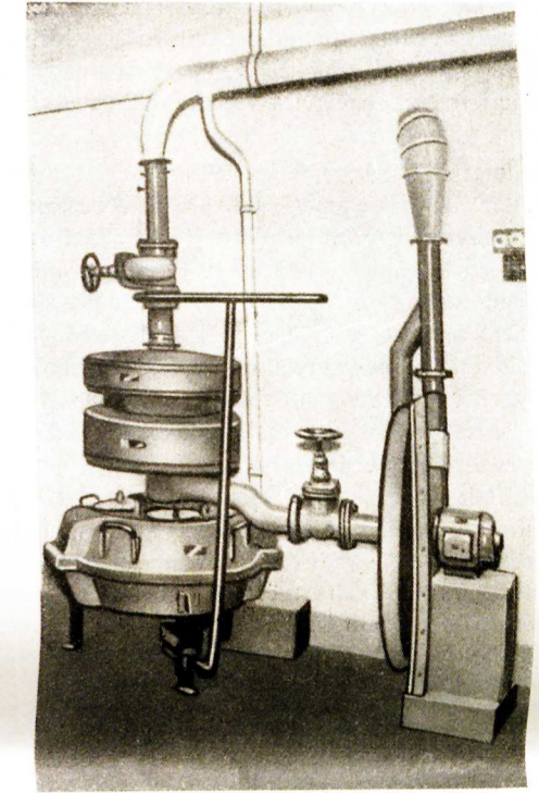
Szab. Auer-óvóhelyszellőztető M. R. 1200 (részben keresztmetszetben).
