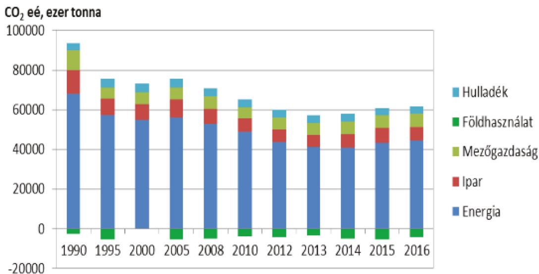
13. ábra. Az üvegházhatású gázok kibocsátása és elnyelése (erdeink évente átlagosan több mint 3 millió tonna szén-dioxidot kötnek meg), CO 2 -egyenérték gigagrammban (kilotonna), a jelölt években ágazatonként Magyarországon 26
