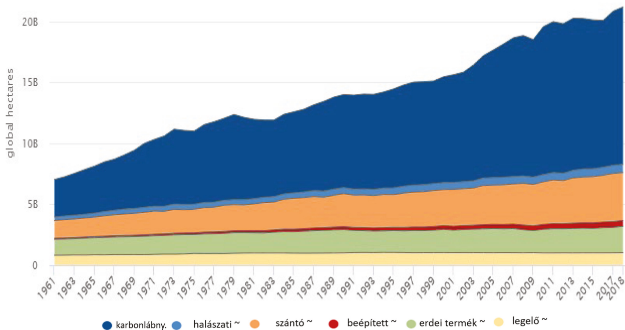
6. ábra. Az emberiség ökológiai lábnyoma összetételének változása (Global Footprint Network, 2020)
