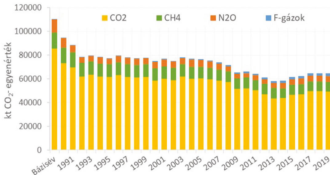
12. ábra. Az üvegházhatású gázok kibocsátása Magyarországon, CO 2 egyenérték gigagrammban (kilotonna), a jelölt években (Forrás: OMSZ)
