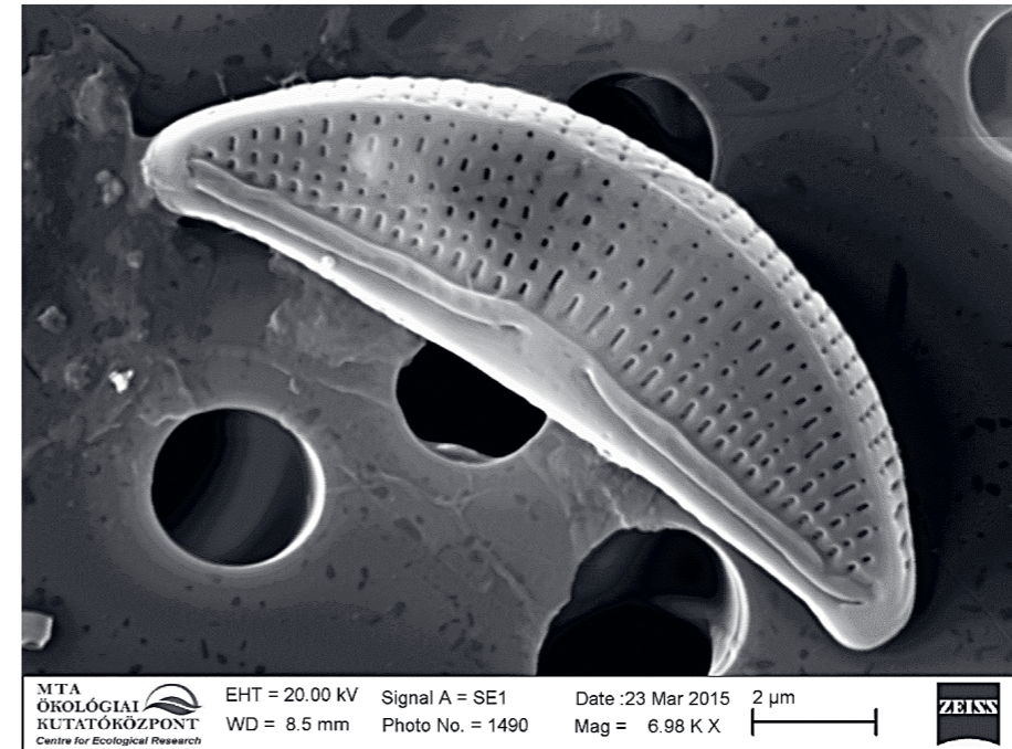
Halamphora dominici pásztázó elektronmikroszkópos képe
