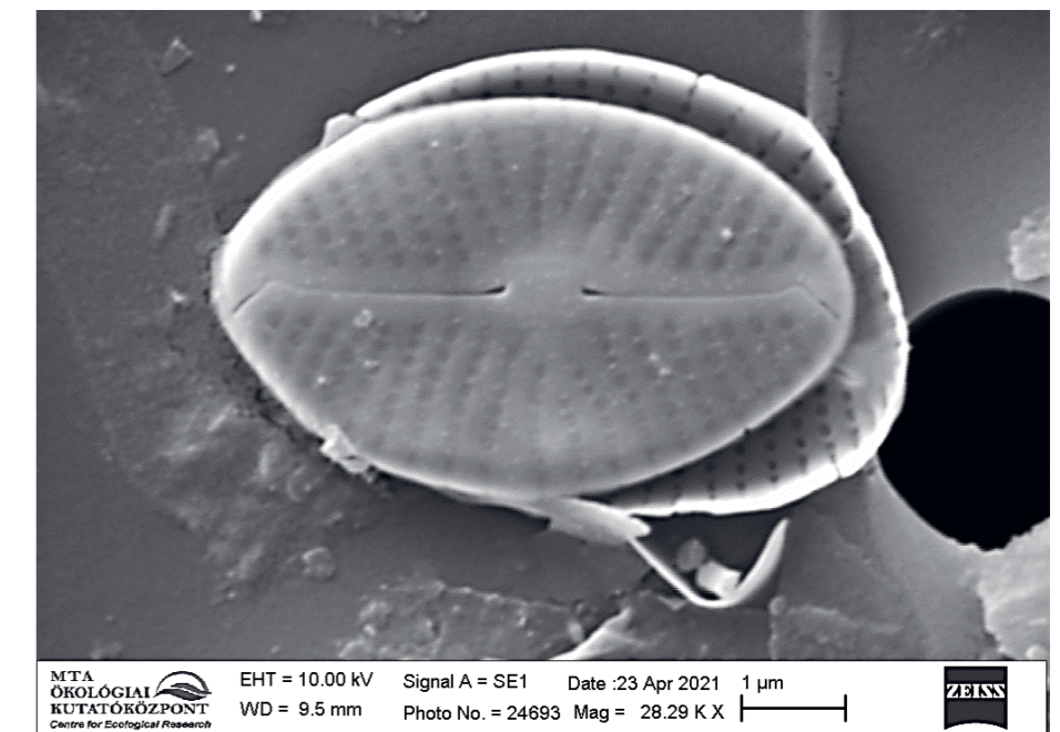
Mayamaea ectorii pásztázó elektronmikroszkópos képe
