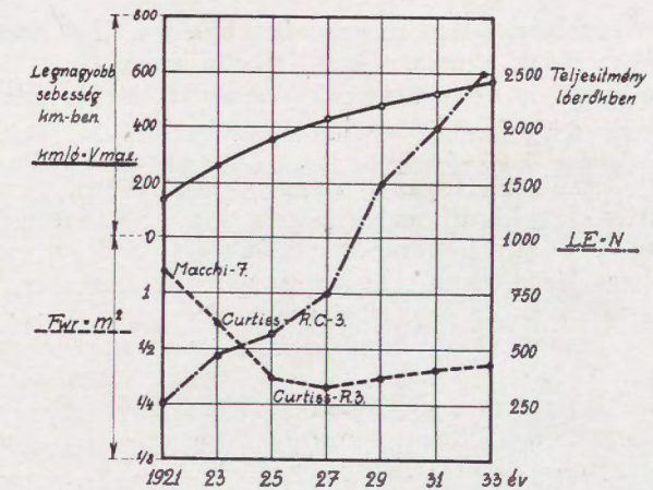
Repülőgép teljesítmény fejlődése az utóbbi években.
