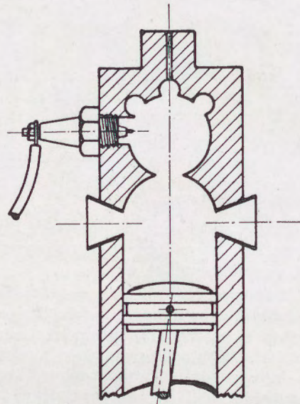
E.J.J. típusú egyhengeres repülőmotor.
