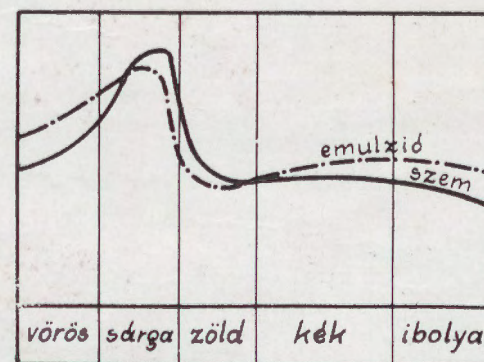
c) A panchromatikus emulzió és a szem érzékenységi görbéje.
