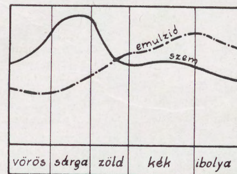
a) Az extra-rapid emulzió és a szem érzékenységi görbéje.
