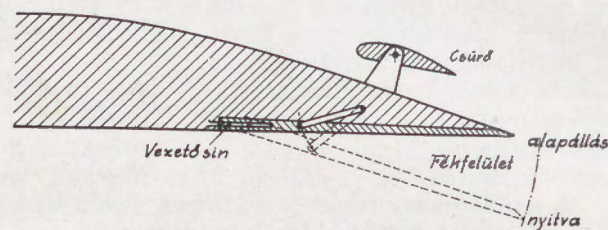
Két különböző fékfelület megoldás.
