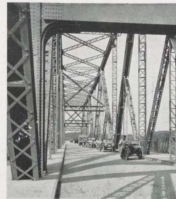
Gk. kiképzésű aks-ok a dunaföldvári hídon (1934).
