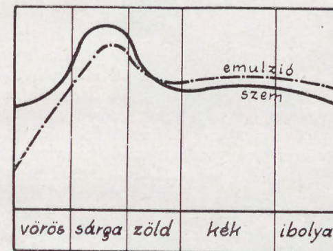
b) Orthochromatikus emulzió és a szem érzékenységi görbéje.
