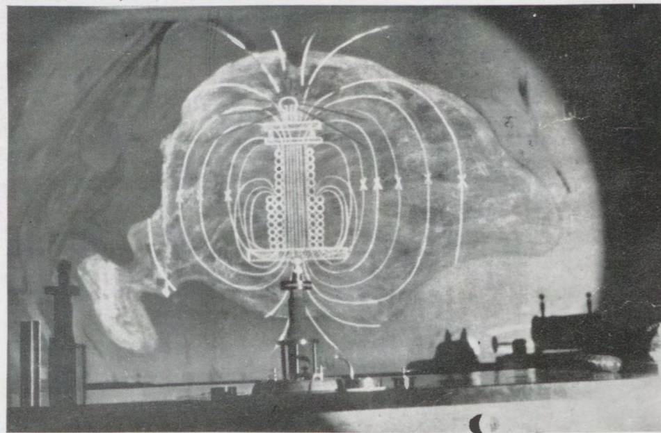
THOMSON-FÉLE KISÉRLET.
