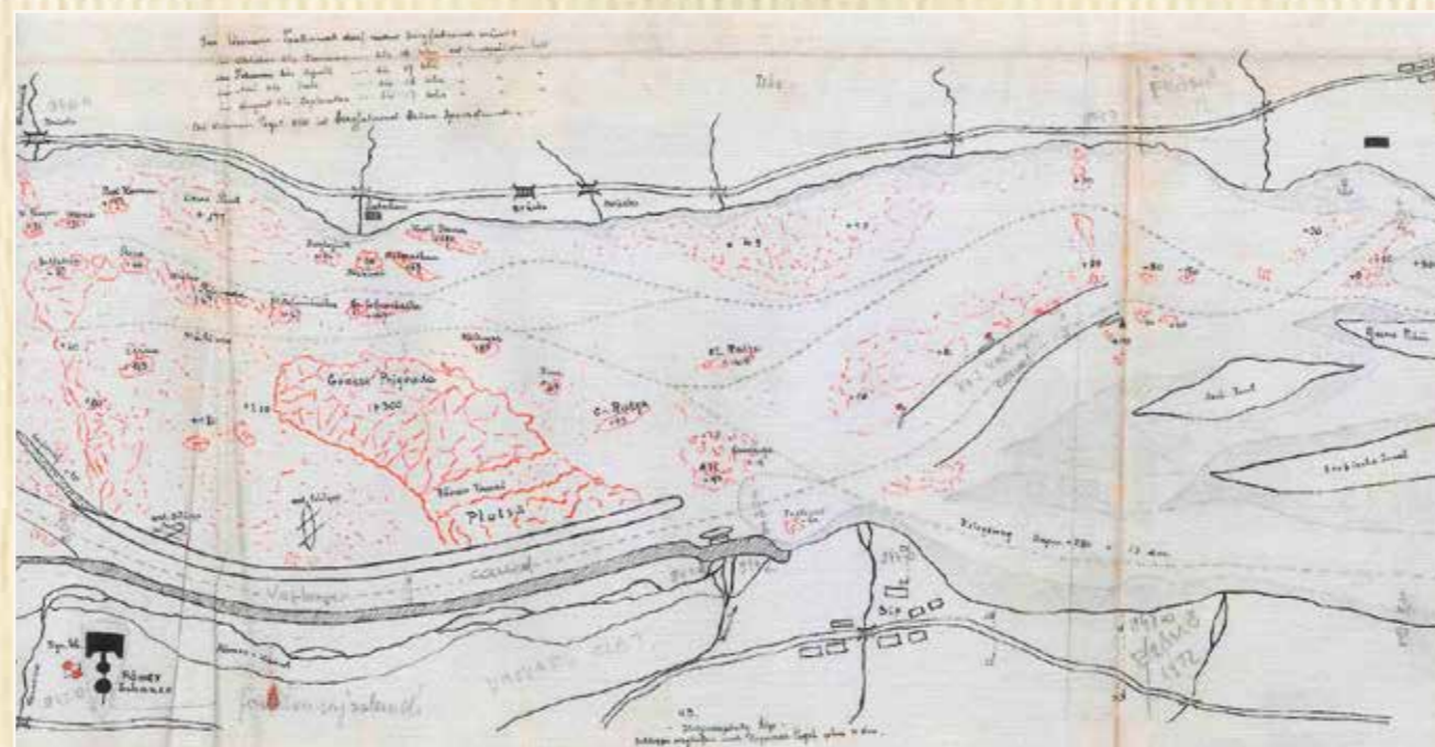
Az építendő meder nyomvonalának térképe
