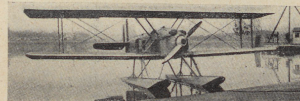
Egy Navy „DT-4” típusú univerzális hidroplán, melyet az amerikaiak leginkább torpedóvetésre és bombázásra használnak
