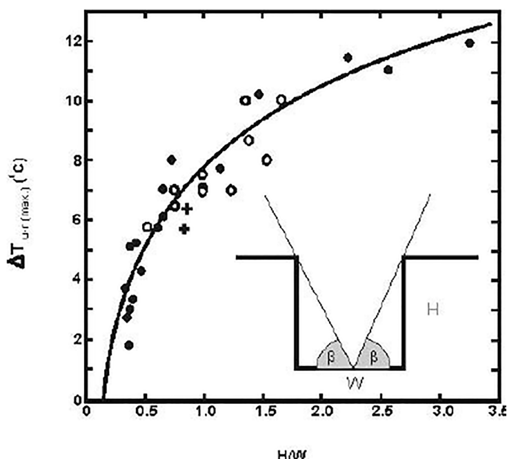
1. ábra. A városi hősziget maximum hőmérsékletének ( \Delta T ) függése az épületmagasság/utcaszélesség ( H/W ) hányadostól
