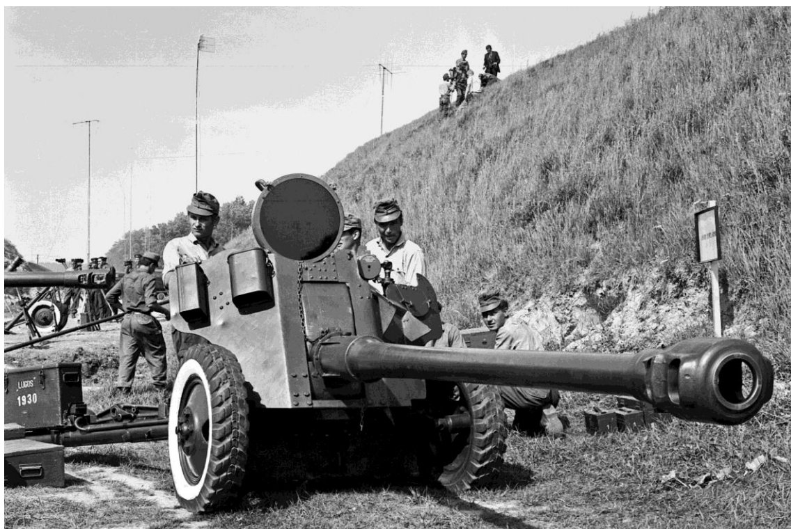
29. kép 85 mm-es D-44 páncéltörő ágyú „N” változat
