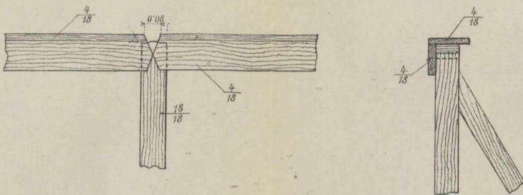
Geländer mit Gelenksverbindung.
