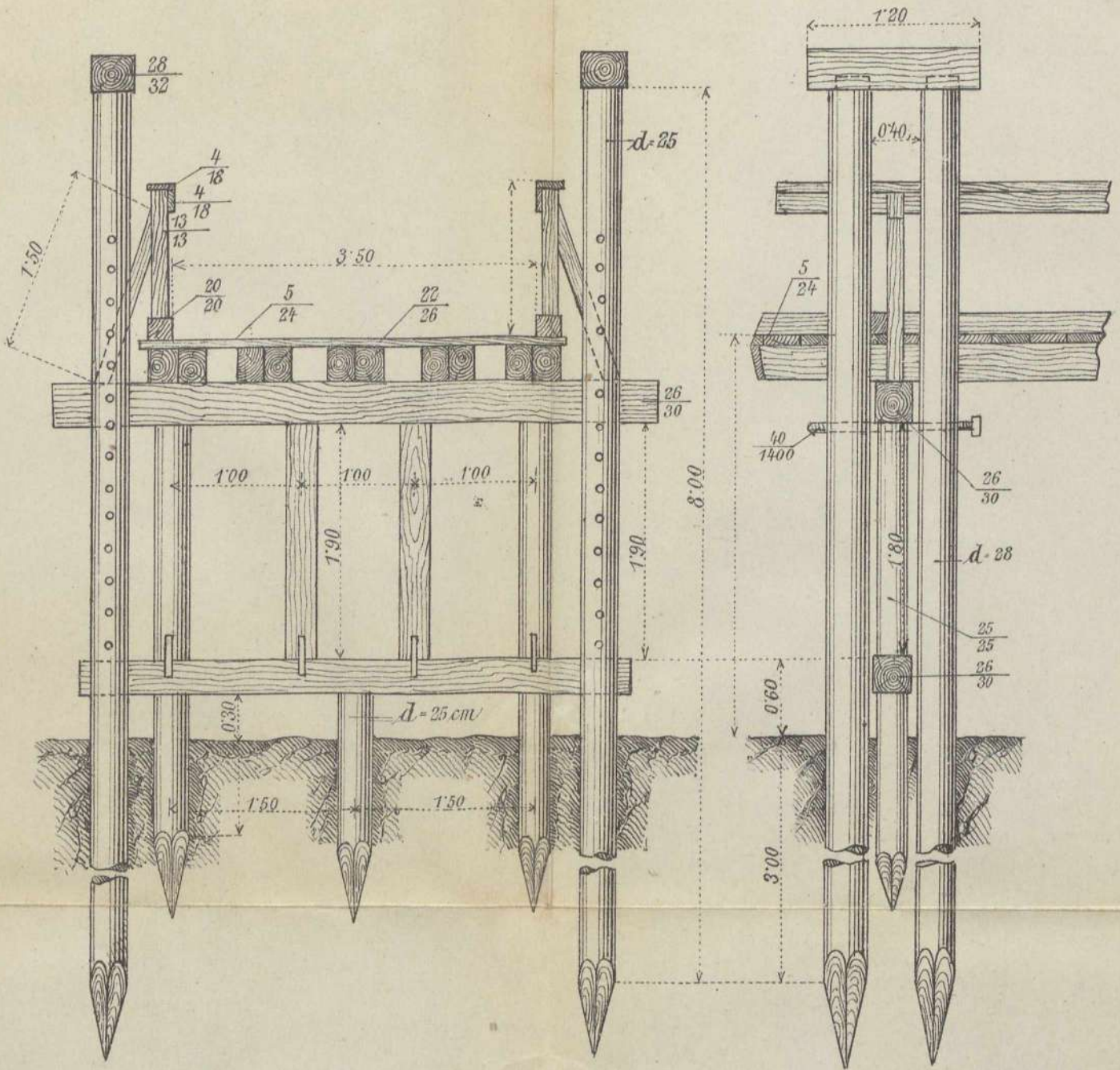
Geländer mit Gelenksverbindung.
