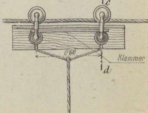
Gleitschlitten mit 2 Messingrollen. Längenschnitt a-b.
