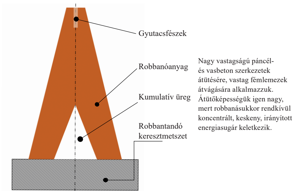
7.13. ábra Kumulatív töltet
