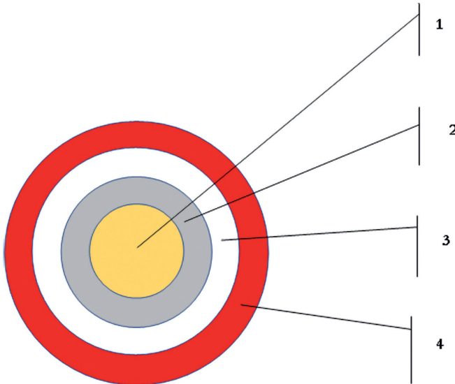
7.18. ábra Robbanó gyújtózsín
