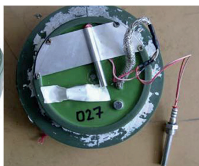
7.4. ábra HAKEG-2 gyújtó
