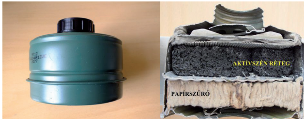
8.10. ábra 93M szűrőbetét
