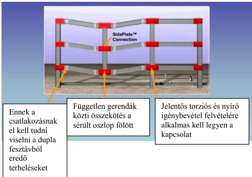
24. sz. ábra. A kieső oszlop terheit átveszik a szomszédos, oldallemezzel megerősített oszlopok (forrás: http://sideplate.com/tech_papers.pdf 2010. 02.14.)
