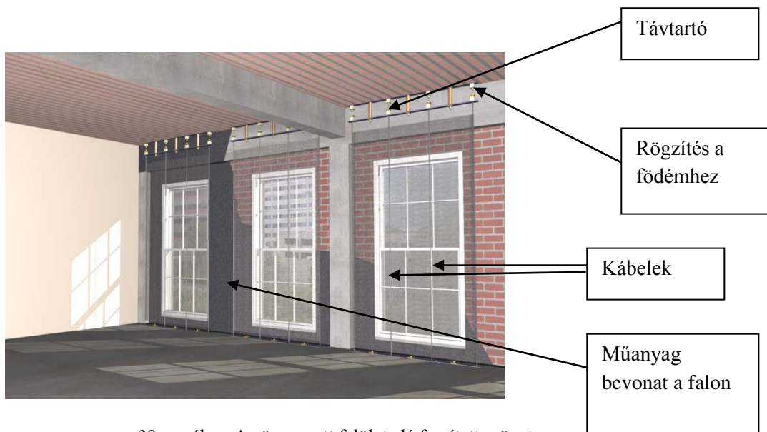
39. sz. ábra. Az üvegezett felület elé feszített szövet (forrás: http://www.kcse.com/pdfs/P-01-32_f.pdf 2011. 05.05)
