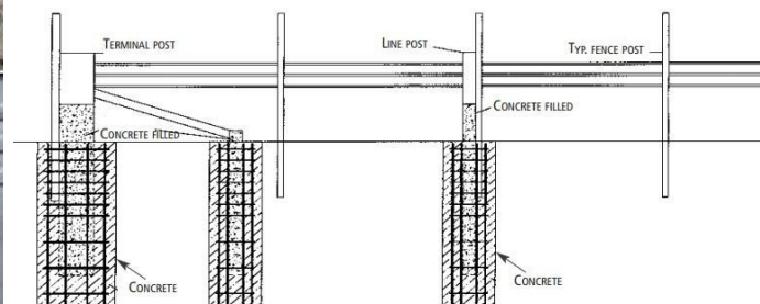
49. sz. ábra. A kis alapozási mélységet igénylő kerítés 1 méteren belül megállítja a teherautót (forrás: http://productsearch.bdonline.co.uk/HS-Jackson-&-Son-crash-rated-fencing-file014966.pdf 2010.07.13.)
