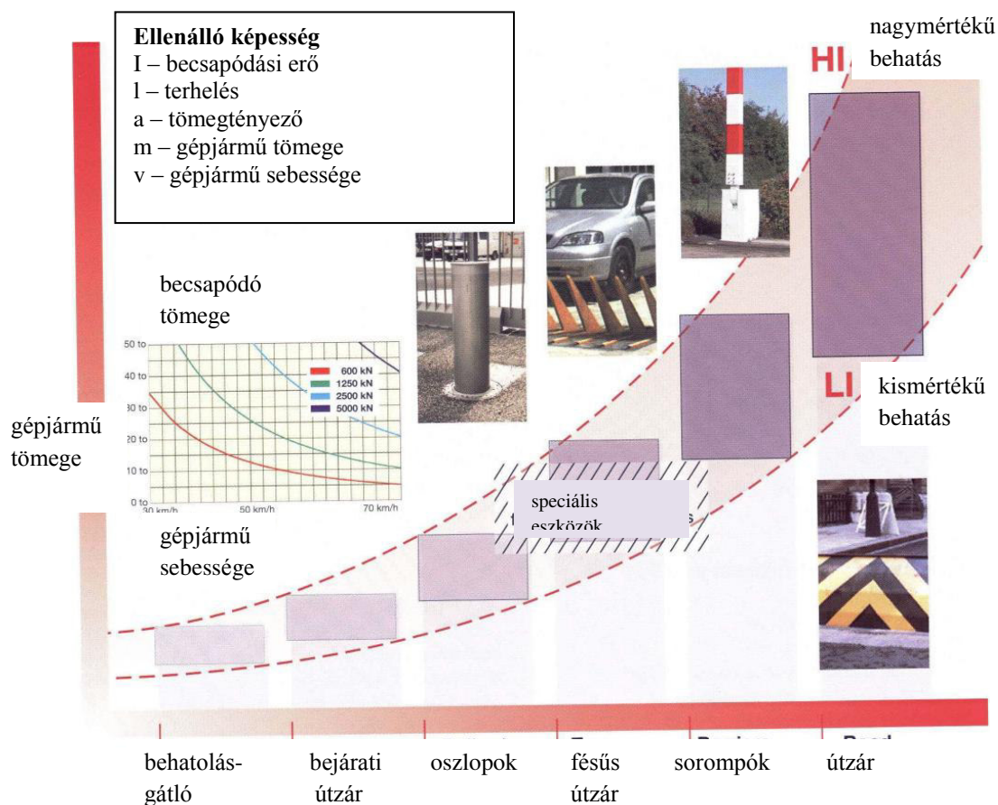
53. sz. ábra. A mechanikai eszközök tárháza (forrás: http://www.gunnebo.com/hu/products/Pages/default.aspx 2010.12.25)
