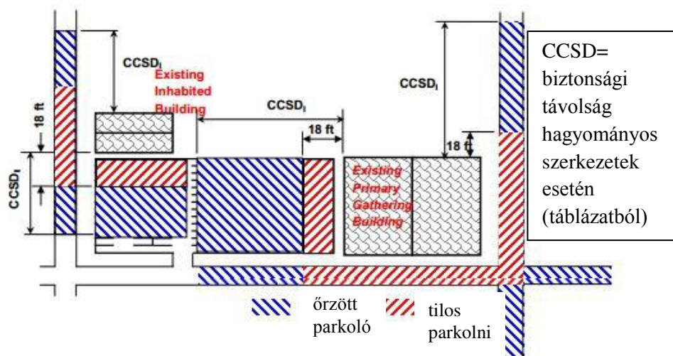
20. sz. ábra. Kerítés nélküli terület (forrás: http://www.wbdg.org/ccb/DOD/UFC/ufc_4_010_01.pdf 2012.02.19.)
