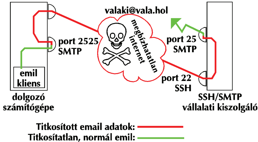
12. ábra SMTP továbbítás SSH alagúton
