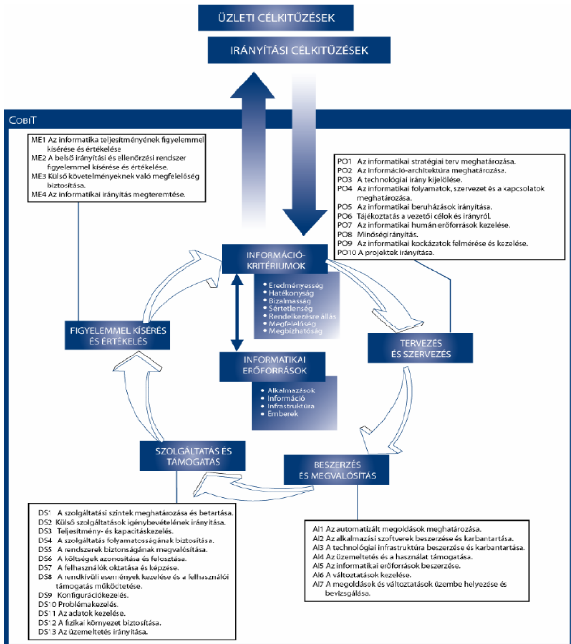
8. ábra Az általános COBIT keretrendszer (Forrás: (ISACA Budapest Chapter, 2011))
